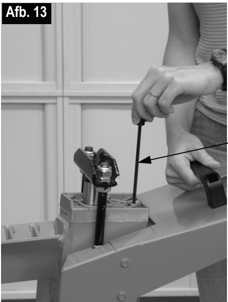
Oliepeilstaaf
